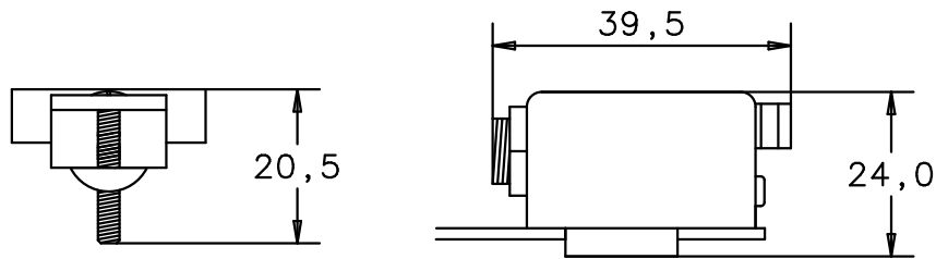
Seitenansicht von links side view left
