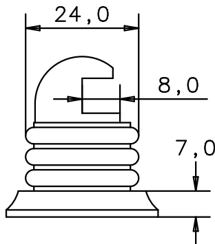
Seitenansicht von links side view left
