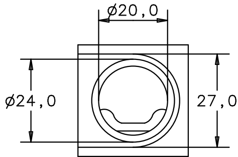
Draufsicht top view
