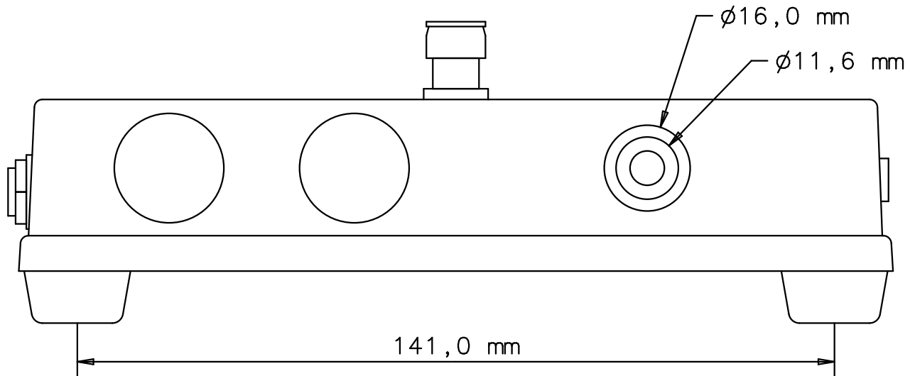
Rückansicht back view
