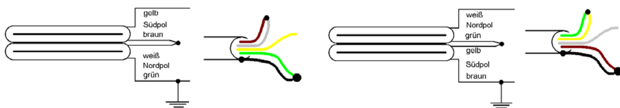
Serienschaltung
