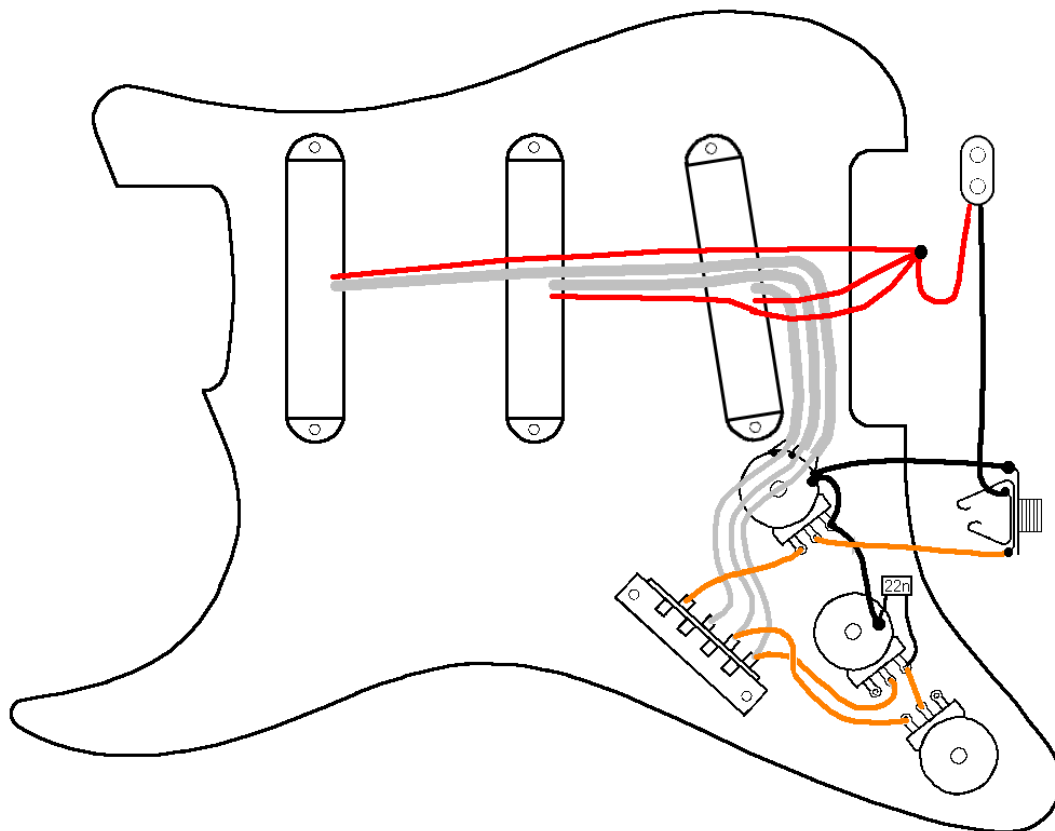
„Stratocaster“-Verdrahtung
