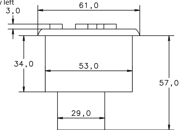
Seitenansicht von links side view left
