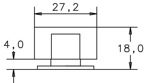
Seitenansicht von links side view left
