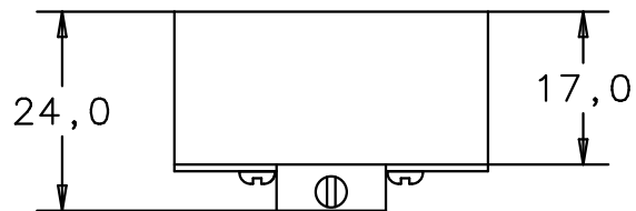
Seitenansicht von links side view left
