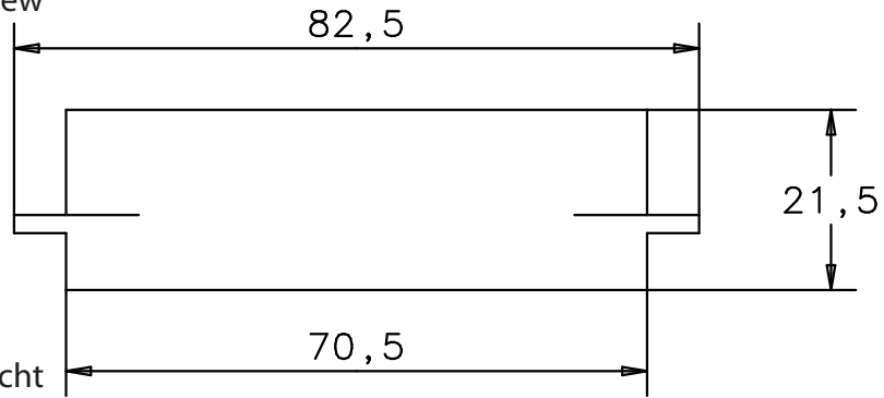
Vorderansicht front view
