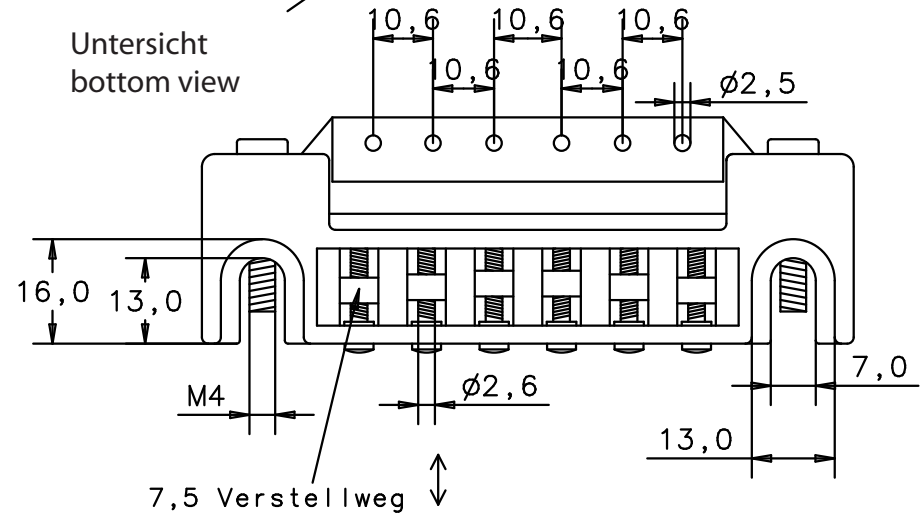
Einschlagmutter insert
