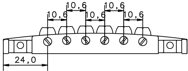
Draufsicht top view
