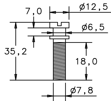
Höhenverstellungsschraube level adjustable screw
