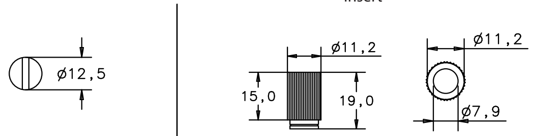
Einschlagmutter insert
