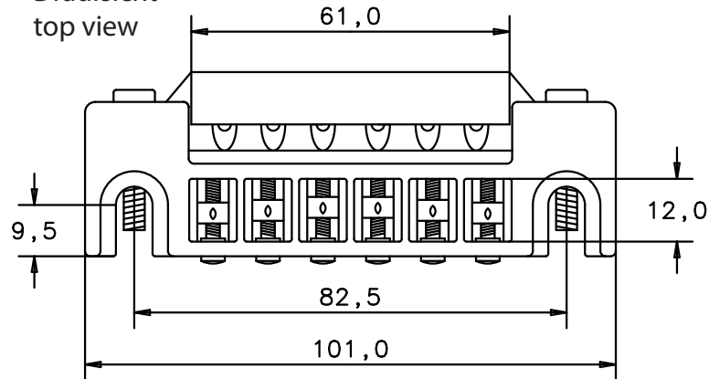
Höhenverstellungsschraube level adjustable screw
