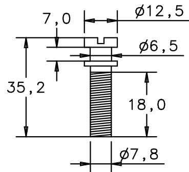
Höhenverstellerschraube level adjustable screw
