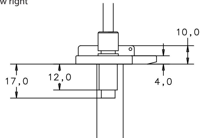
Seitenansicht von rechts side view right
