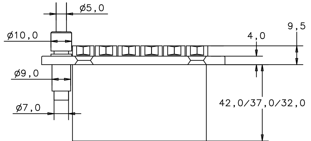
Rückansicht back view
