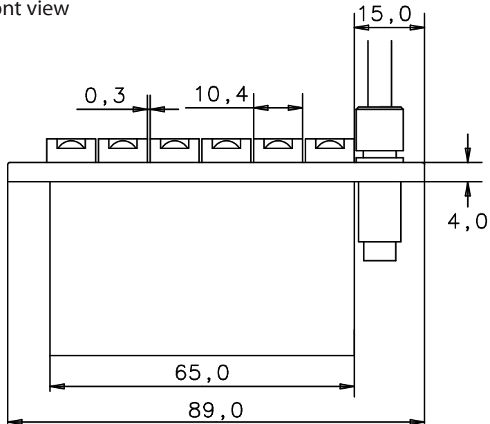
Vorderansicht front view
